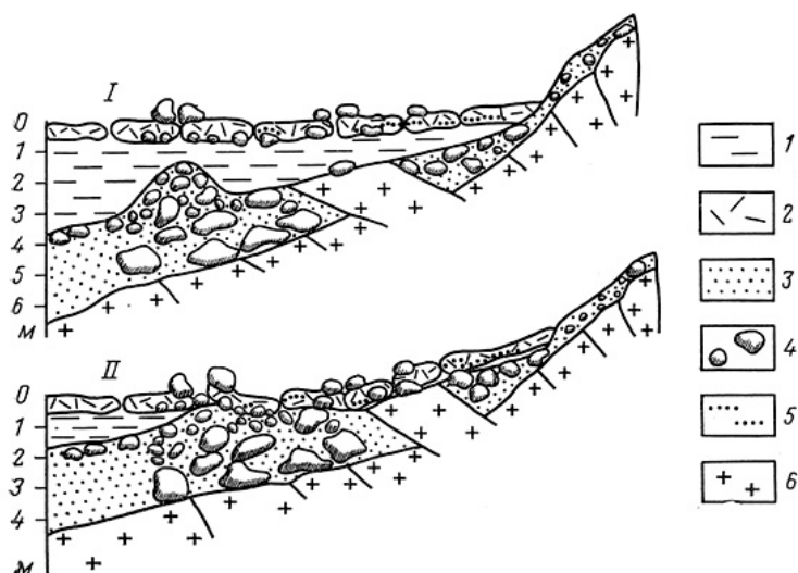
Рис. 1. Строение и схема загрузки припая Кандалакшского залива терригенным материалом: 1 — уровень моря при приливе (I) и отливе (II), 2 — припайный лед, 3 — пески, 4 — валуны и глыбы, 5 — галька и гравий, 6 — коренные породы
