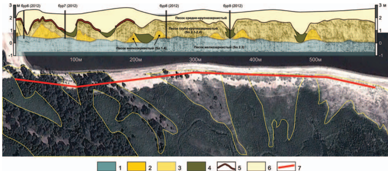
Рис. 3. Интерпретация георадарного профиля ГПРБИ 11-12, секущего серию кулисообразных кос
