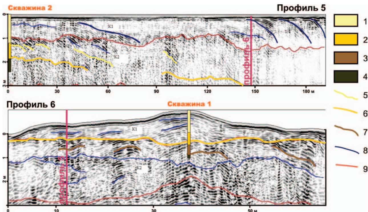
Рис. 4. Георадарные профили через дистальный край песчаной косы
