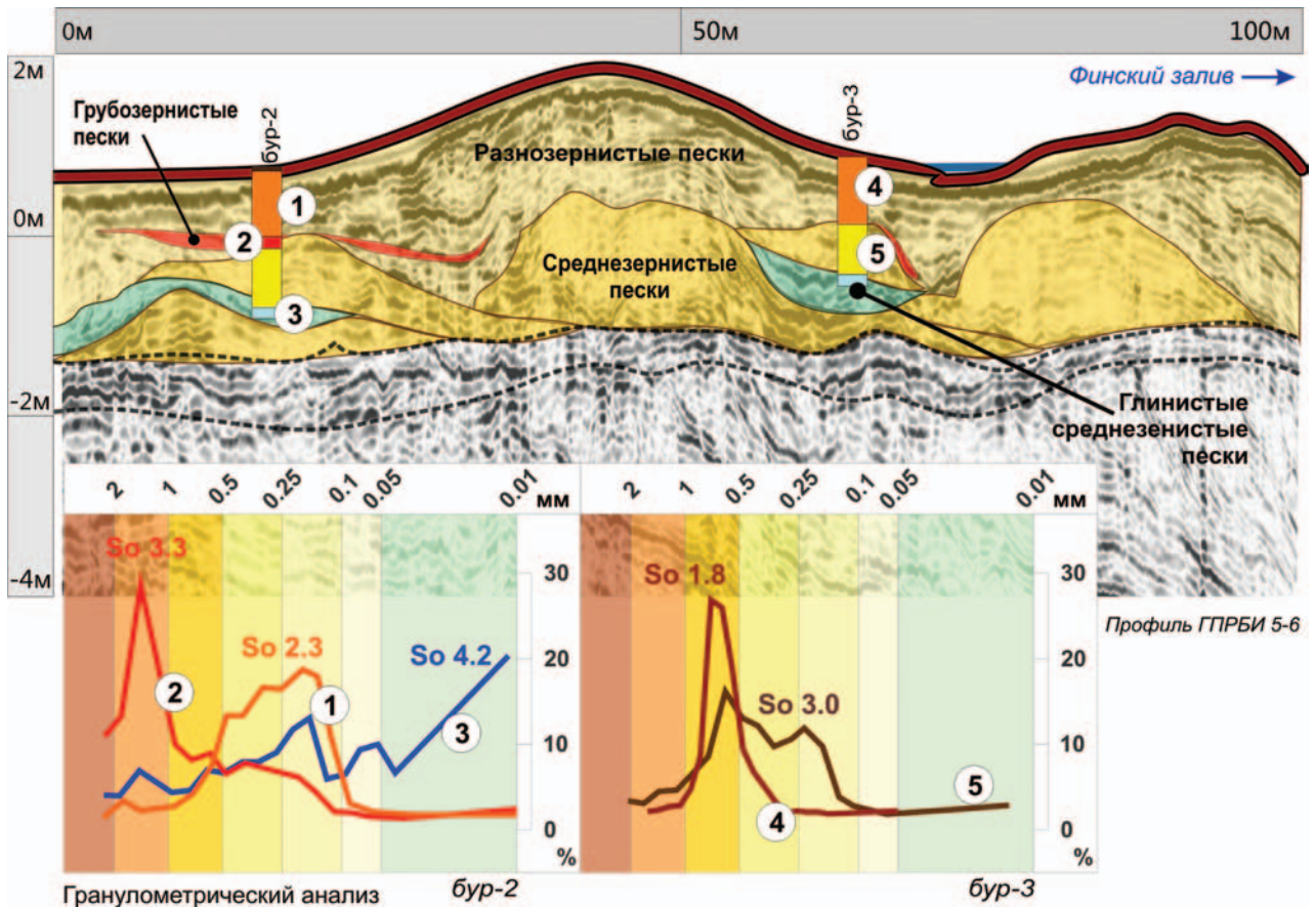
Рис. 2. Интерпретация профиля георадара ГПРБИ 5-6
