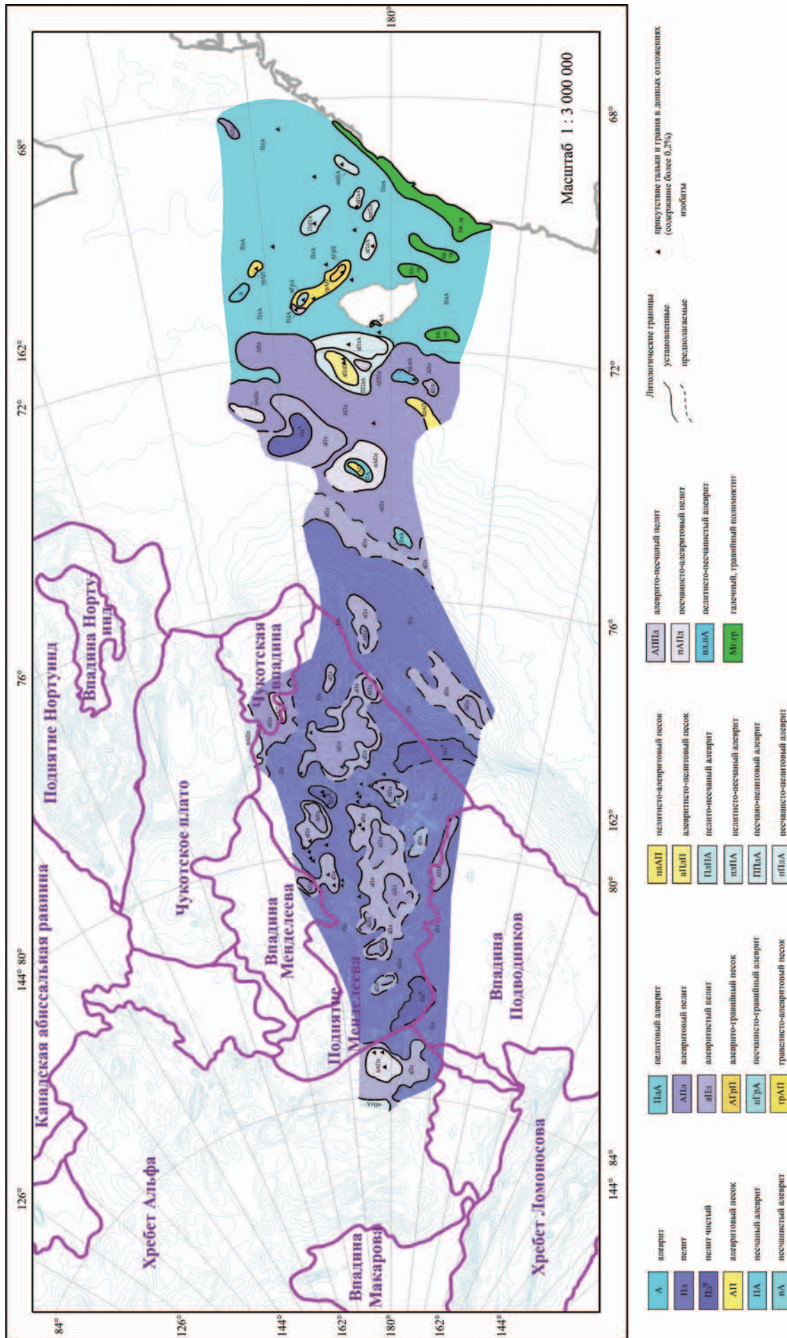
Рис. 8. Литологическая карта донных осадков поднятия Менделеева и сопряжённых структур
